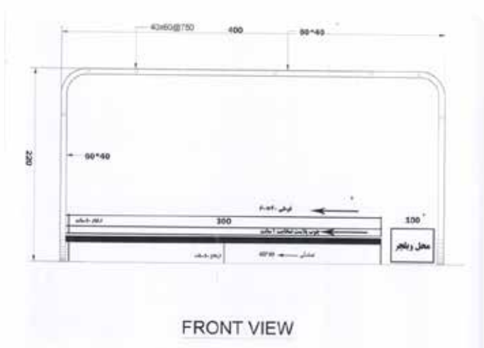
یک نمونه طراحی سرپناه مناسب معلولین.
